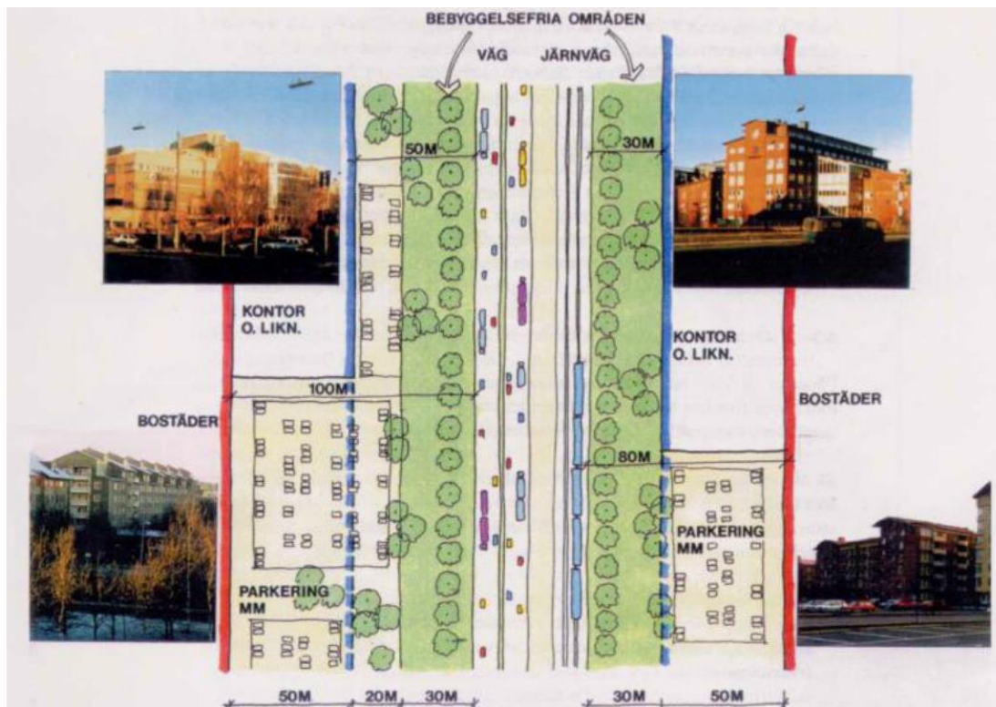
Figur 5. Fysisk ram kring transportleder för farligt gods invid förnyelseområden.
