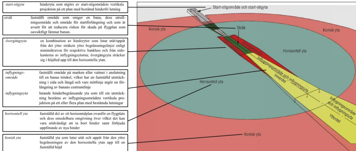
Figur 13. Förklaring och illustration av hinderbegränsade ytor [11].
