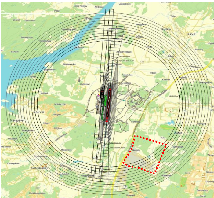
Figur 12. Hinderbegränsade ytor omkring Säve flygplats [10]. Röd markering anger ungefärlig placering inom vilket studerat detaljplan är placerat.
